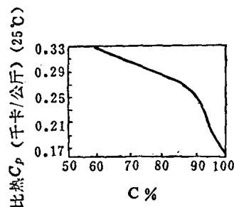
图 1-5 炭化程度与比热关系
