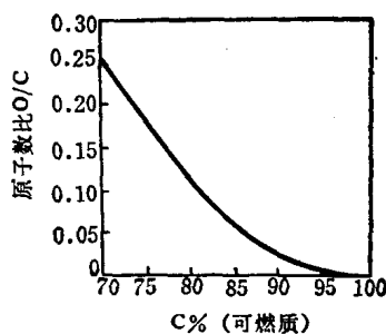
图 1-2 煤的含氧量与炭化程度的关系
