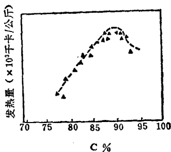
图 1-4 炭化程度与发热量的关系
