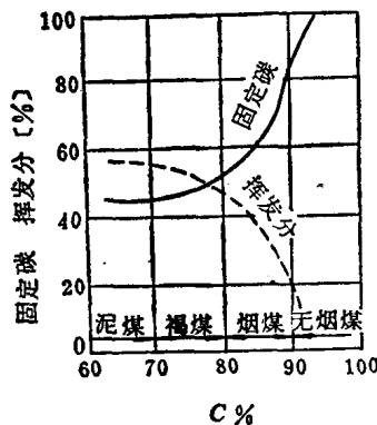
图 1-3 固定碳以及挥发分与炭化程度关系
