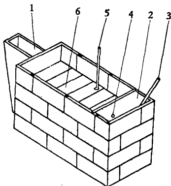
图 1 自动升降水压沼气池外形
