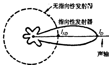
图 0-3 发射指向性图案
