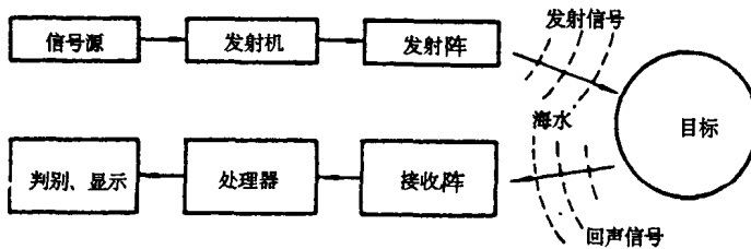
图 0-1 主动声纳信息流程示意图
