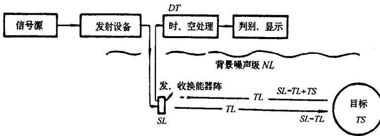
图0-4 主动声纳信号强度变化示意图
