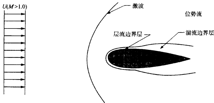
图 1-7 超声速绕流
