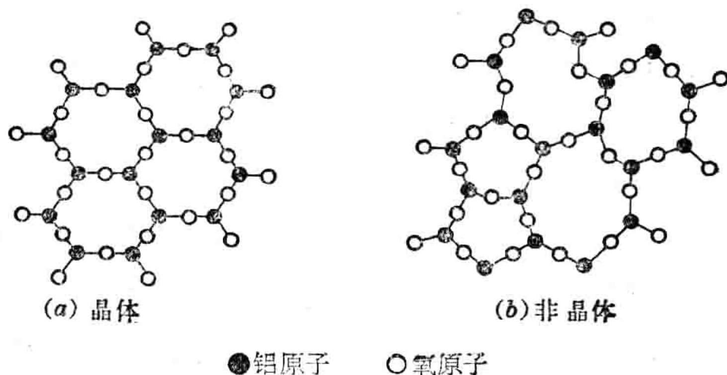
图 1-2 固体氧化铝中原子的排列(平面图)
