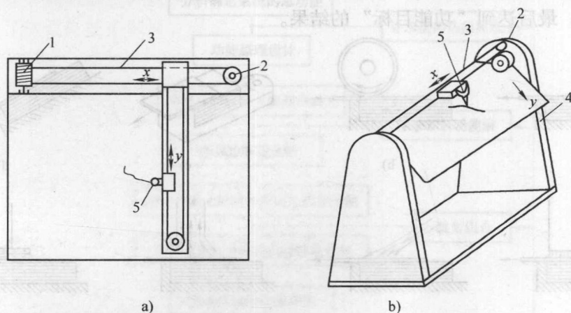
图 2-5 绘图机
