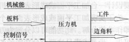
图 2-3 压力机系统的功能分析
