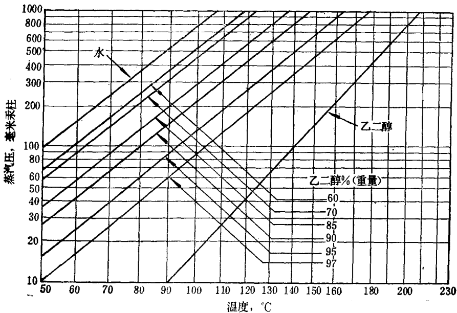
图 5-1 乙二醇水溶液的蒸汽压
