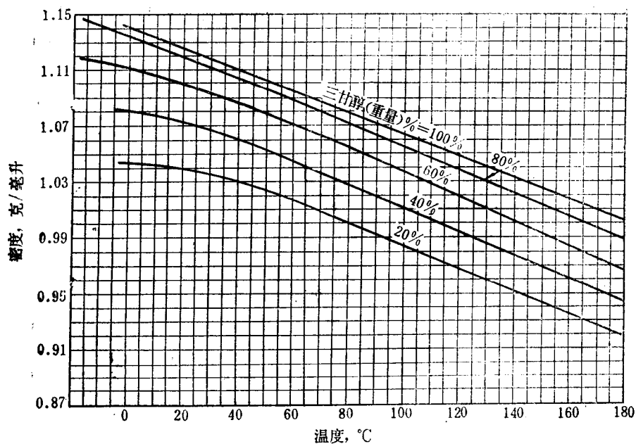
图 5-6 三甘醇水溶液的密度
