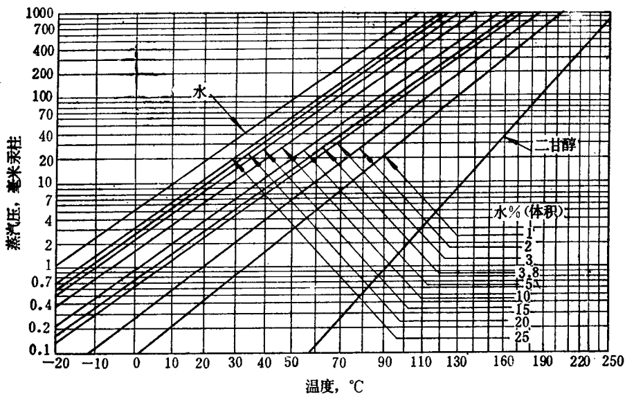
图 5-2 二甘醇水溶液蒸汽压
