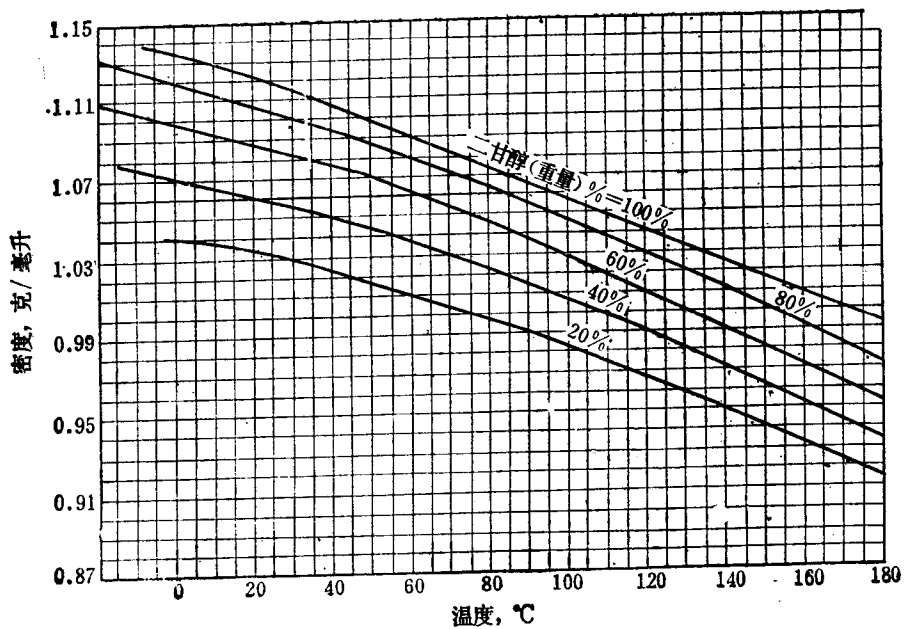
图 5-5 二甘醇水溶液的密度
