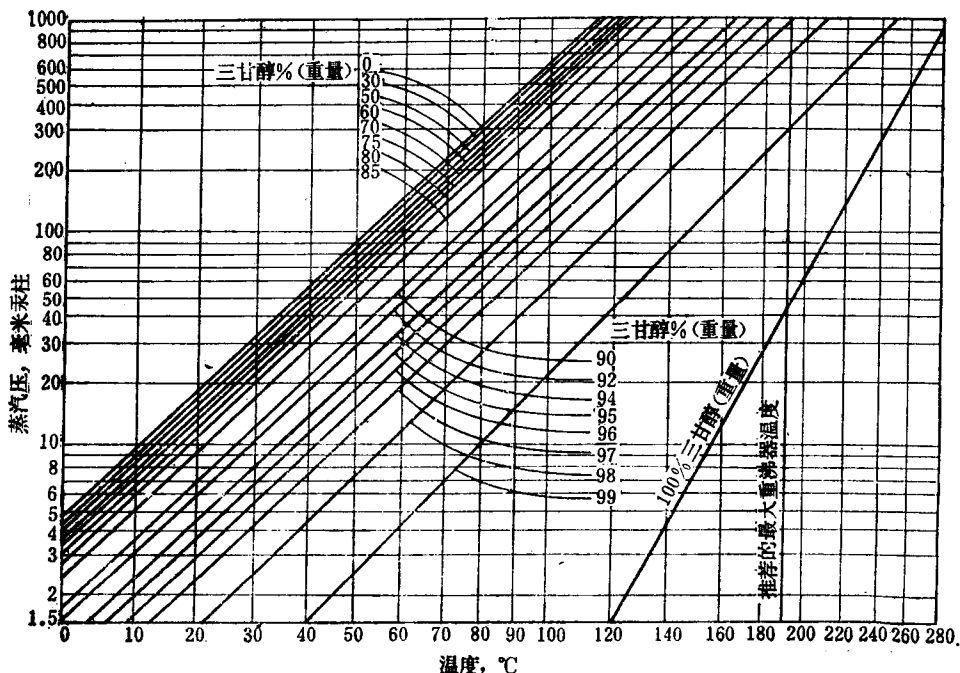
图 5-3 三甘醇水溶液的蒸汽压
