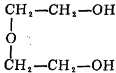
二甘醇
