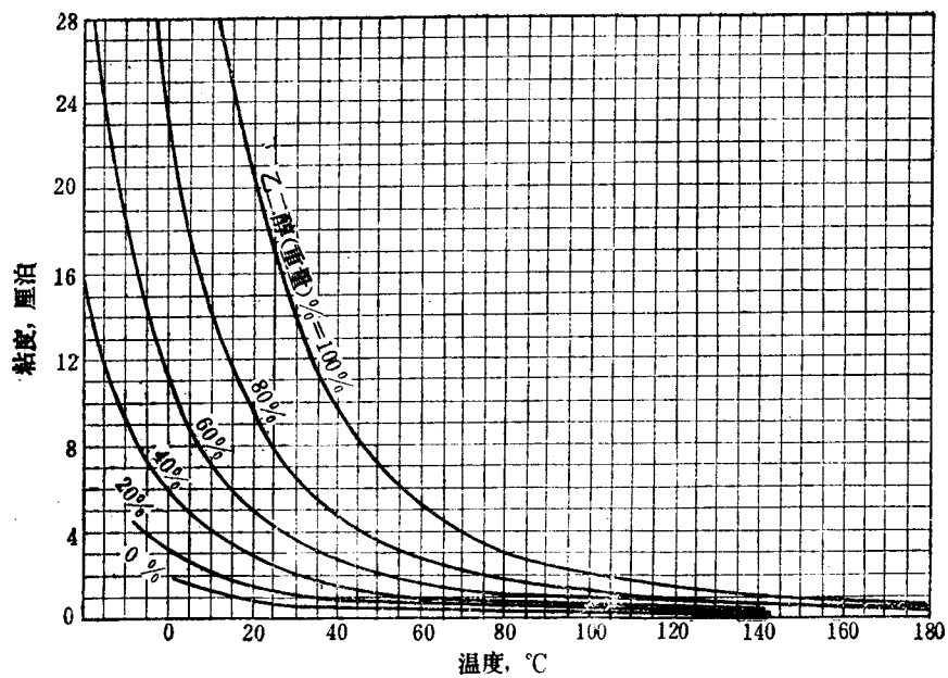
图 5-7 乙二醇水溶液的粘度
