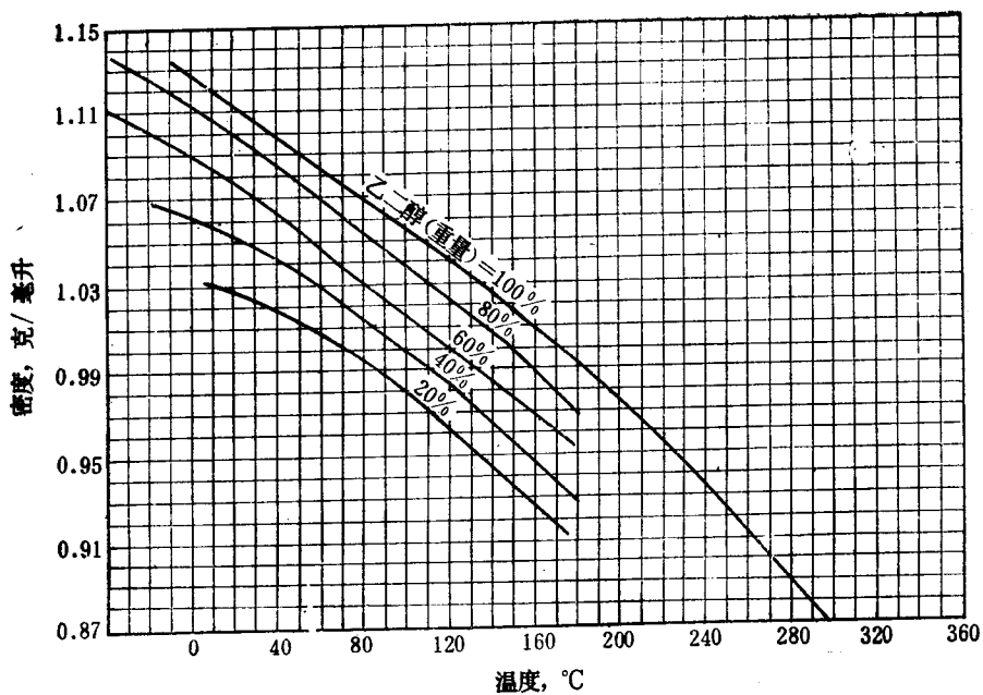
图 5-4 乙二醇水溶液的密度
