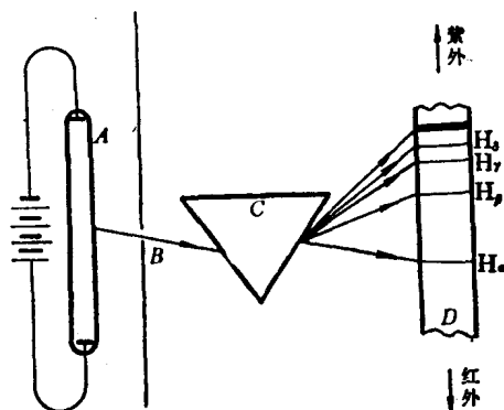
图 1-1 氢发射光谱实验示意图
