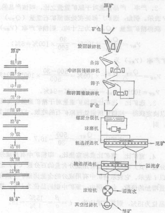
图 0-1 选矿作业的原则流程
