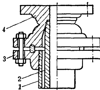
图 1—9 套管头
