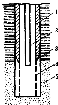
图 1—8 贯眼完成
