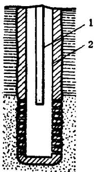
图1—3 射孔完成 1—油管; 2—套管
