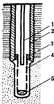
图 1—7 衬管完成
