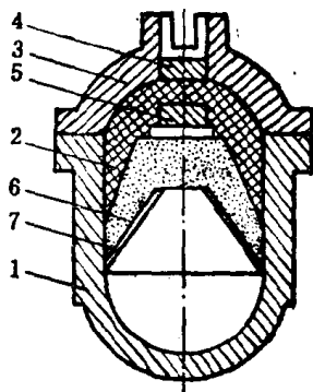
图1—4 聚能喷流射孔器 1—弹壳盖; 2—炸药柱内座; 3— 弹壳底座; 4—铅药饼; 5—起炸药饼; 6—炸药柱; 7—金属锥斗
