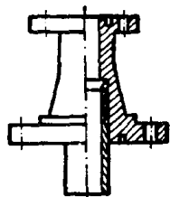
图 1—11 油管头
