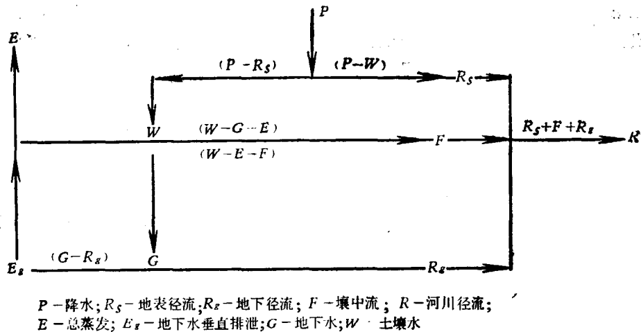
图1 各类水转化关系图
