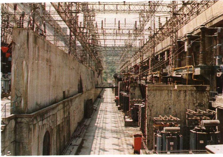
升压变电所
