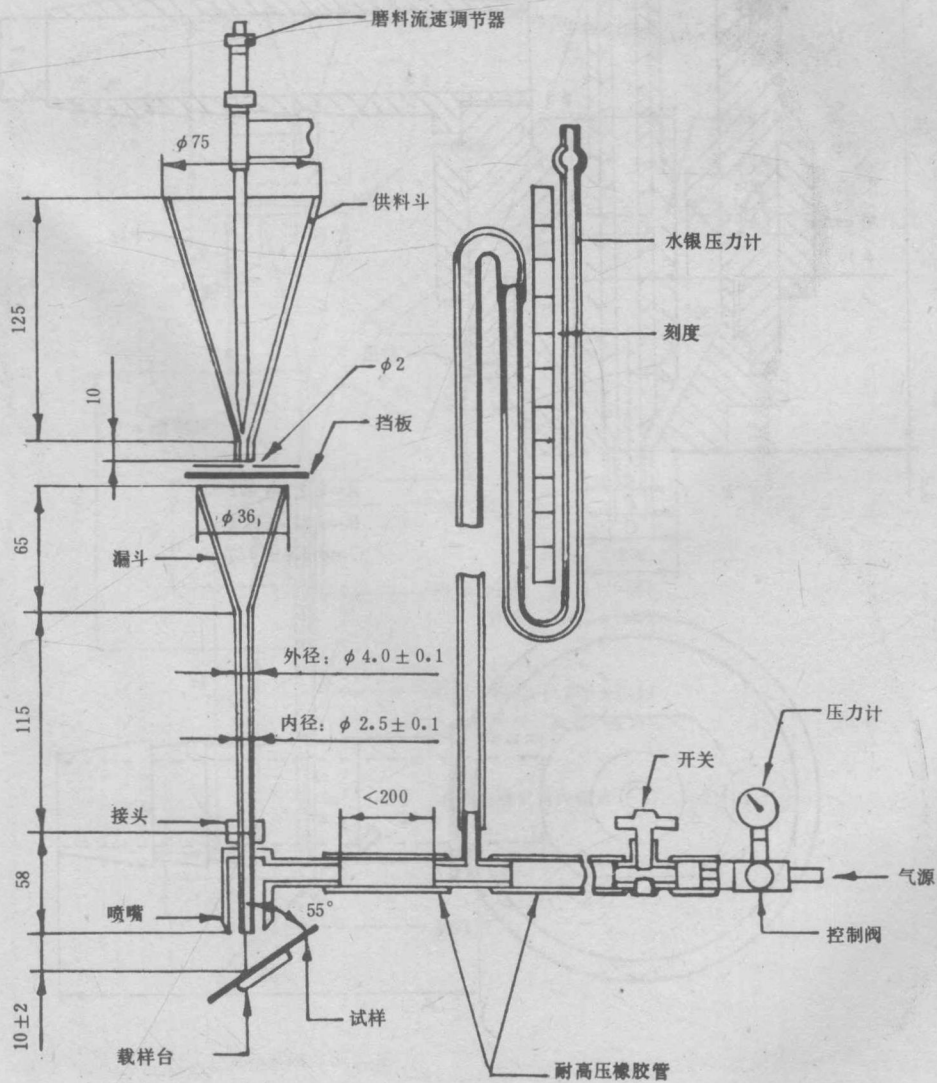
图 A1 喷磨试验仪的基本结构
