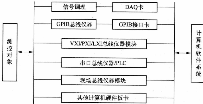
图 1.1 虚拟仪器的硬件结构
