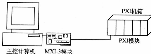
图 1.5 基于 PXI 总线方式的虚拟仪器构成示意图
