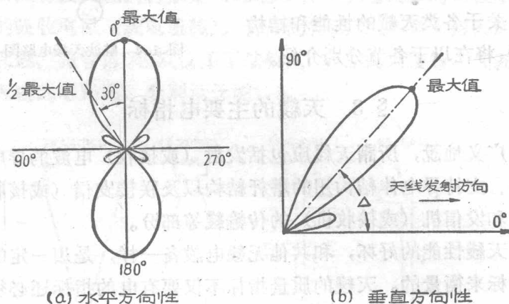
圖 1.5 天綫的方向圖
