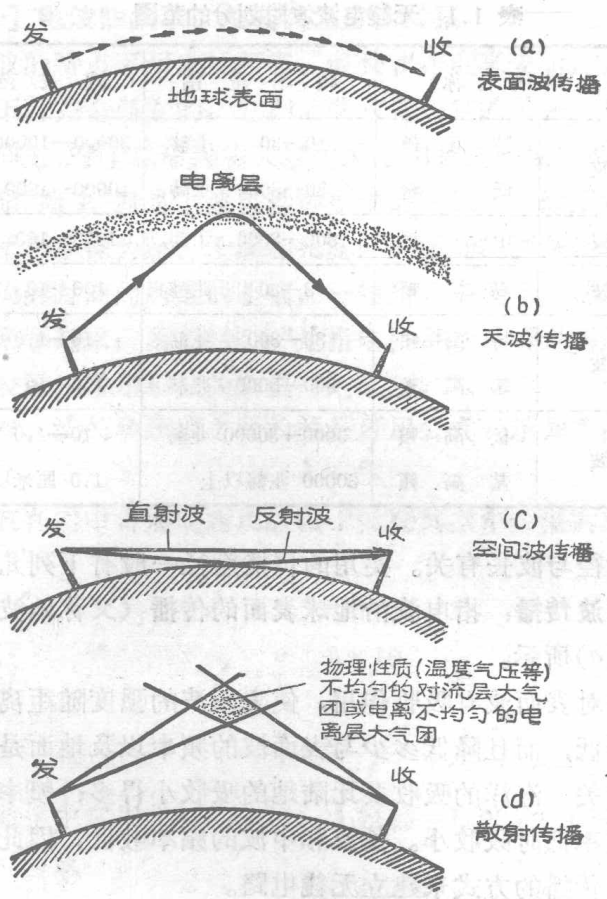
图 1.2 电波传播的几种方式
