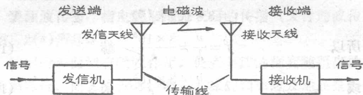
图 1.1 无线电通信工作情况示意图
