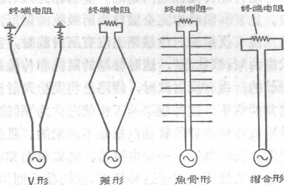
图 1.3 行波天綫电路图
