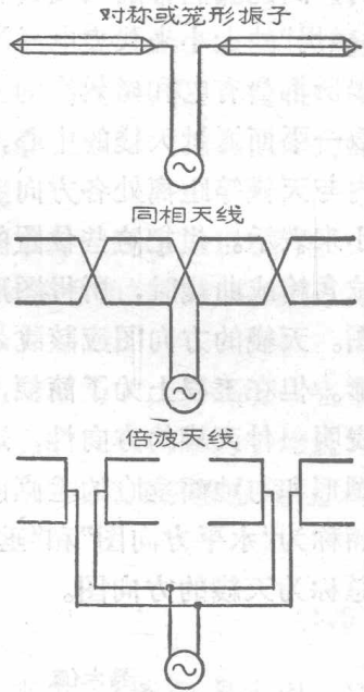
图 1.4 駐波天綫电路图
