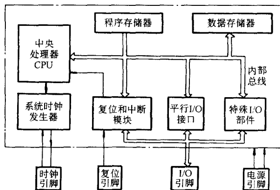
图 1-1 典型的单片机内部结构
