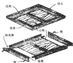
图 1-14 攒边作法
