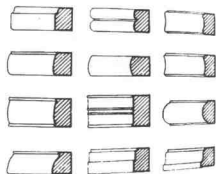
图 1-12 家具腿足断面图
