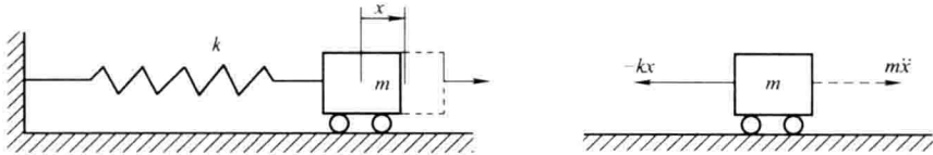
图 1.1 单自由度振动系统的力学模型
