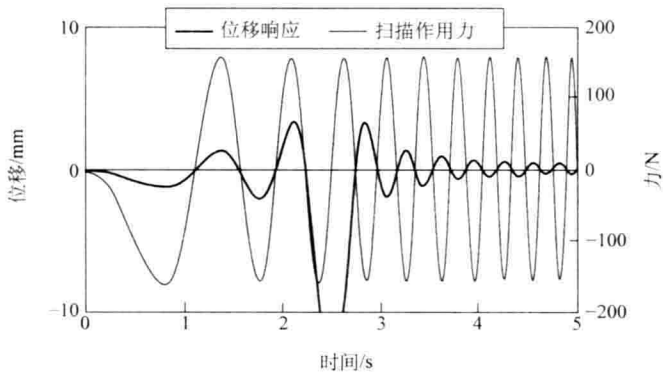
图 1.7 正弦扫描激振时的位移响应及激振力
