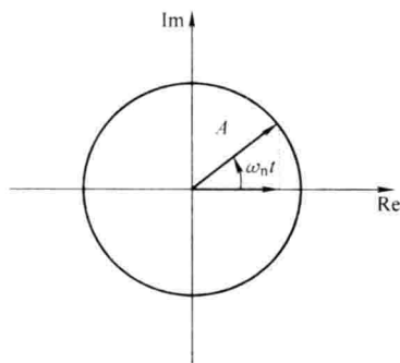
图 1.3 简谐振动的向量表示形式
