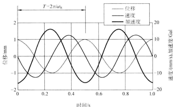
图 1.4 无阻尼单自由度系统的自由振动
