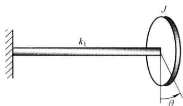
图 1.2 扭转振动系统
