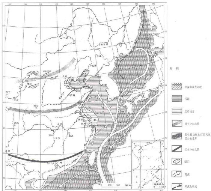
1-1a 晚更新世中国东部环境图。
