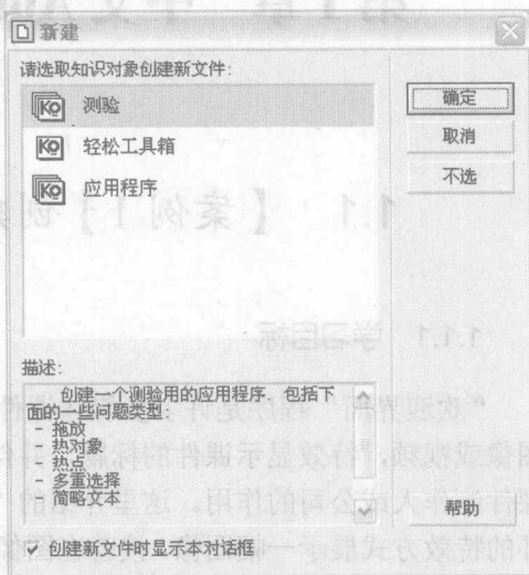
图 1-1-3 “新建”对话框
