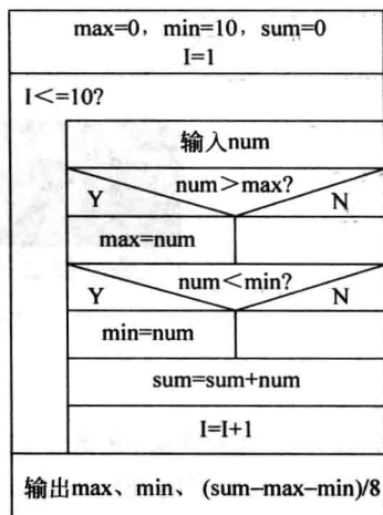
图 1-5 用 N-S 盒图表示的算法
