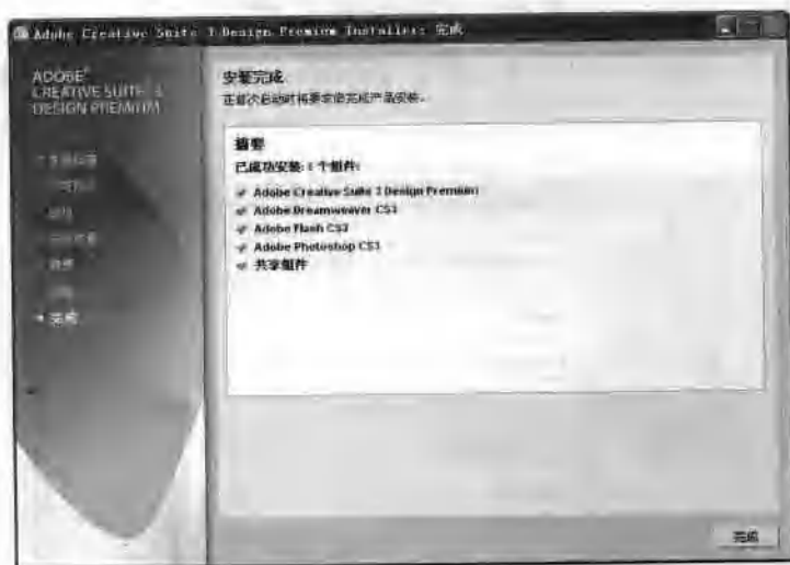
图 1-7 安装完成
