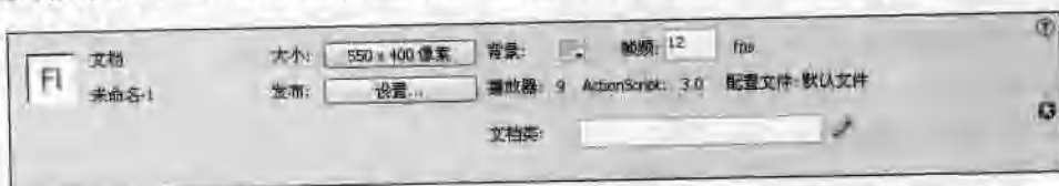
图 1-12 “属性”面板
