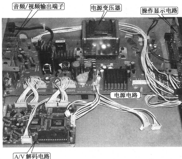
图 1-6 操作显示电路、电源电路、A/V 解码电路和输出端子的连接关系
