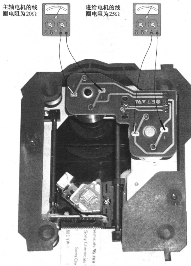
图 1-10 激光头的进给机构
