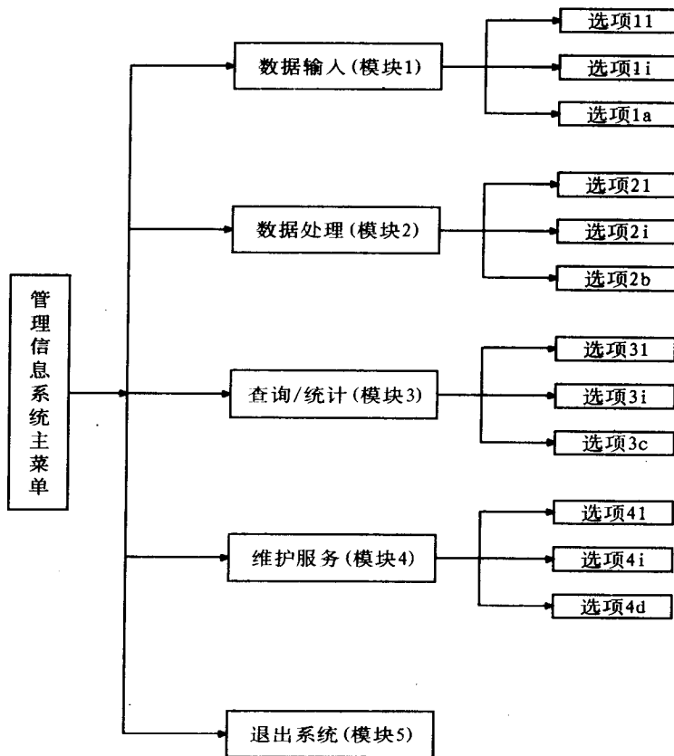
图1-1 管理信息系统程序的结构
