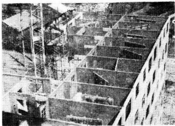
图 4 大模板现浇墙体
