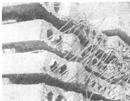
图 6 卡口式预应力钢筋混凝土楼板
