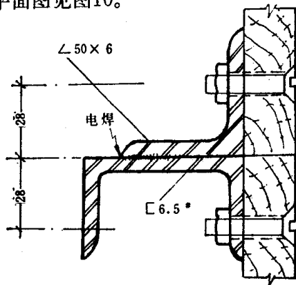
图 9 大模板面板的拼接
