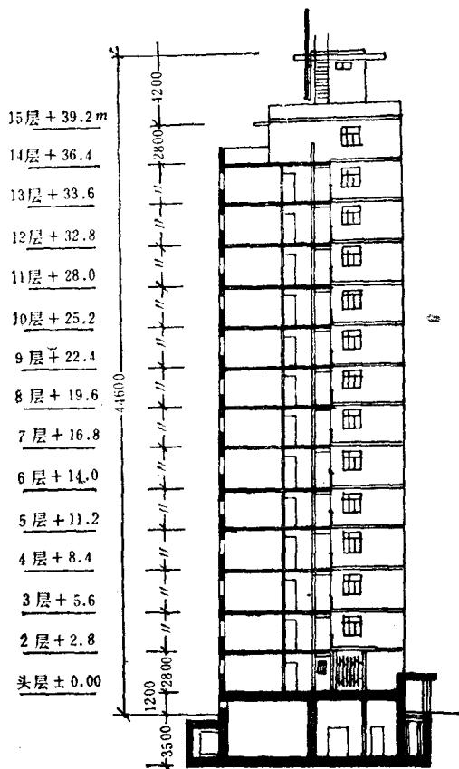
剖面图
