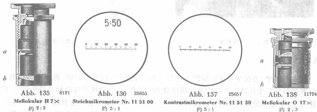
图 2-5 测微目镜
