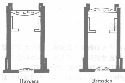
图 2-2 惠更斯目镜和冉斯登目镜的剖面图
