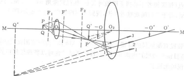
图 2-1 接目镜的放大功能
