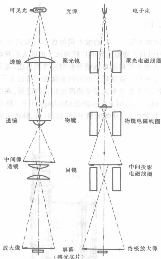
图 1-3 光学显微镜与电子显微镜的物像放大原理和对比示意图
