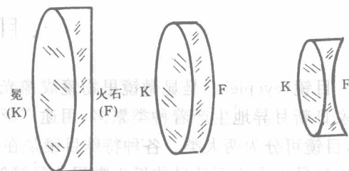
图 2-3 消色差透镜组 (光学玻璃分两大类 1, 冕玻璃 2, 火石玻璃)
