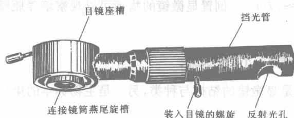
图 1-6 Olympus 厂出产显微镜绘图装置(BH2-DA 型)
