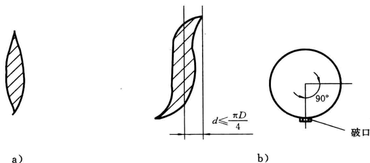
图 1 爆破口形状尺寸
