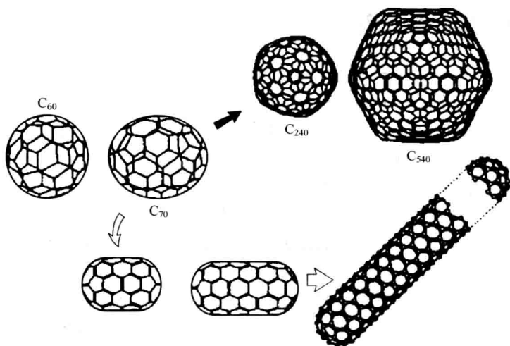
图 1-4 富勒碳的原子结构
