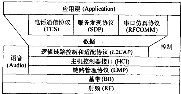
图 1-2 蓝牙协议栈
