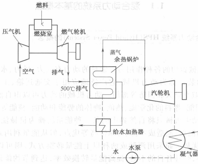
图 1-1 燃气/蒸气混合动力系统组成示意图
