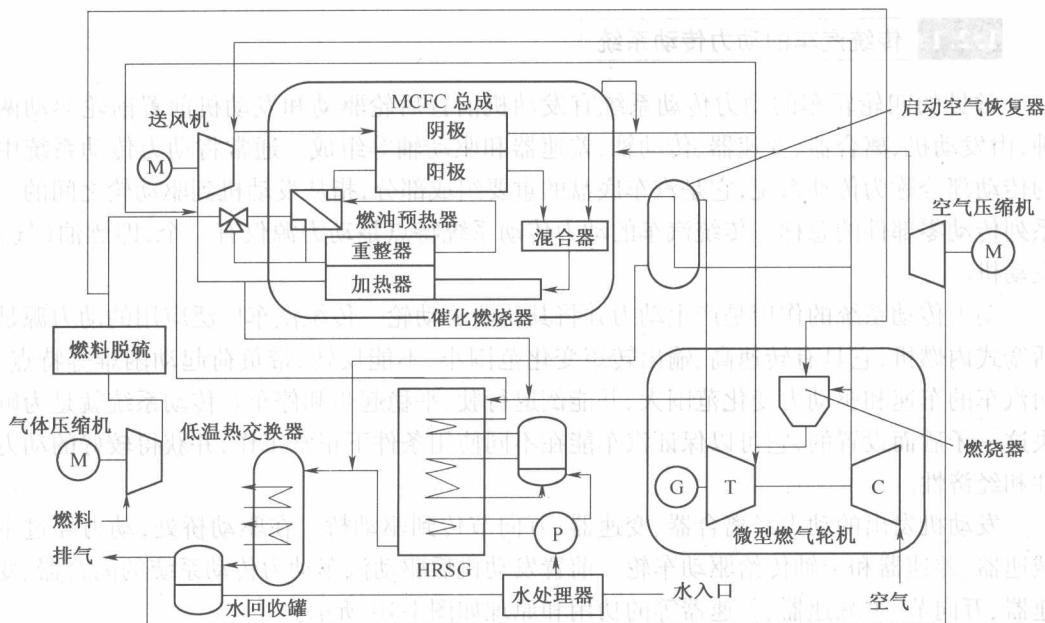
图 1-8 MCFC/MGT 混合系统的工作原理示意图
