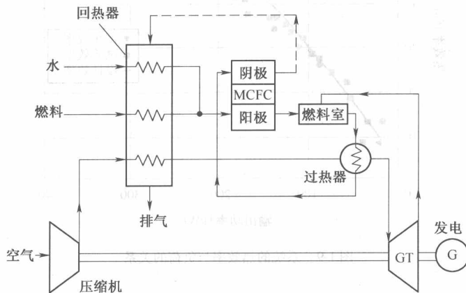
图 1-7 MCFC/GT 系统工作原理示意图
