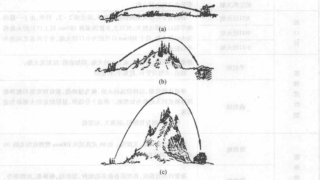
图 2-2 火炮弹道性能示意图 (a) 加农炮; (b) 榴弹炮; (c) 迫击炮。
