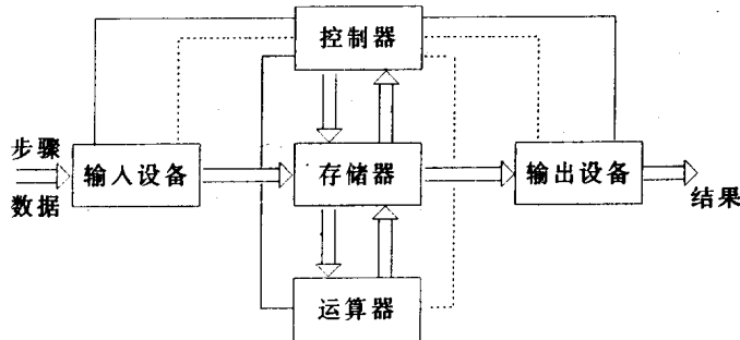
图 1-1 微型计算机的组成框图
