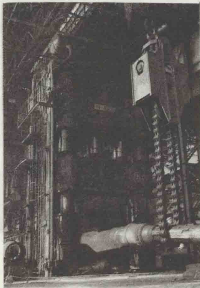
富拉尔基重型机器厂制成 中国第一台万吨水压机。
