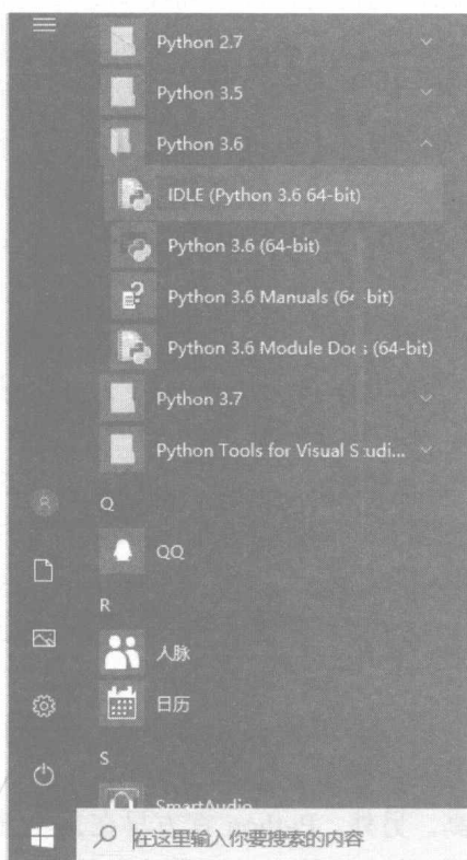
图 1-1 “开始”菜单
