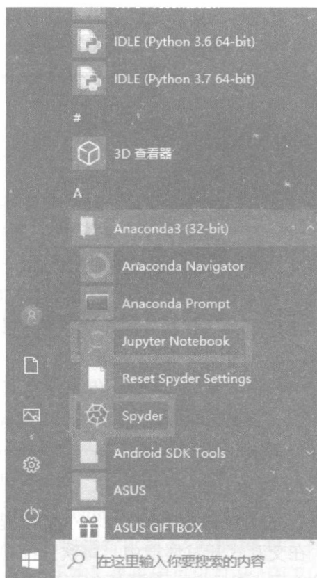
图 1-4 “开始”菜单
