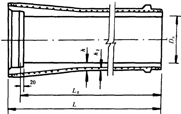
图 1 管子外形
