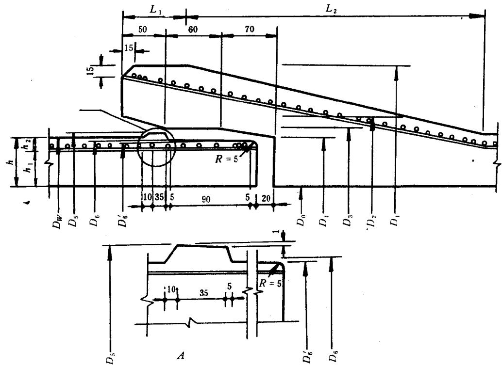
图 2 管子接头
