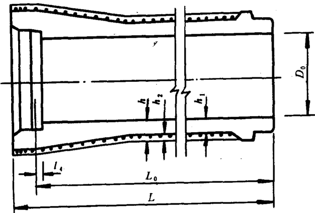
图 1 管子外形
