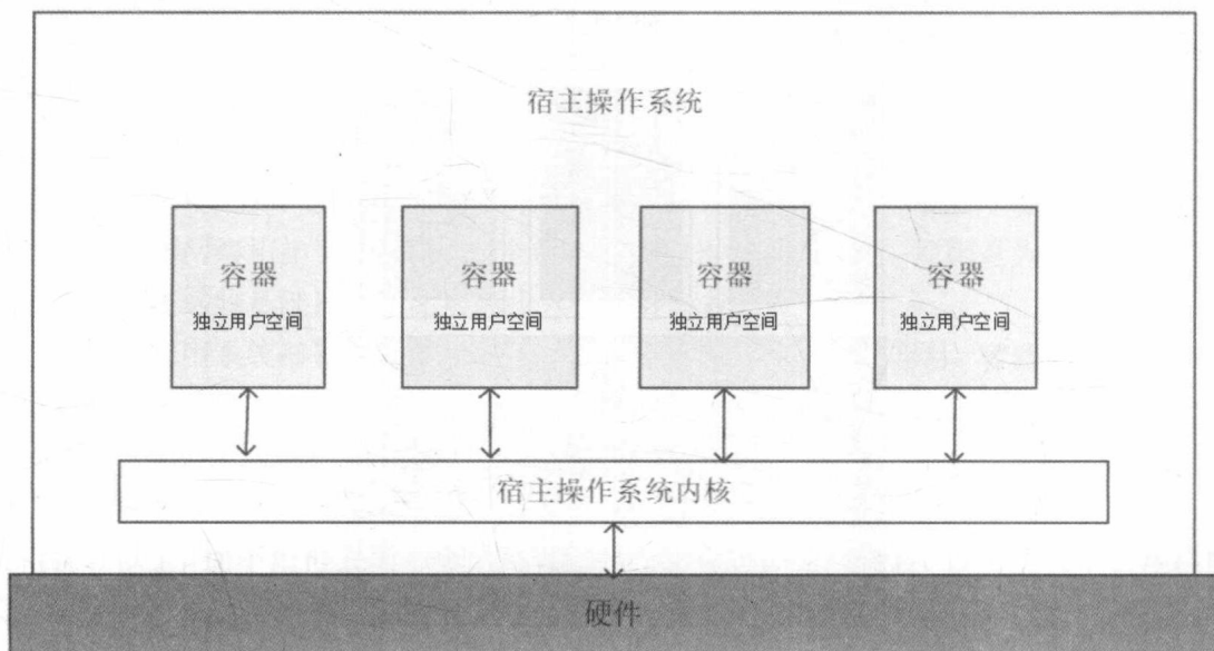
图 1-1 容器架构
