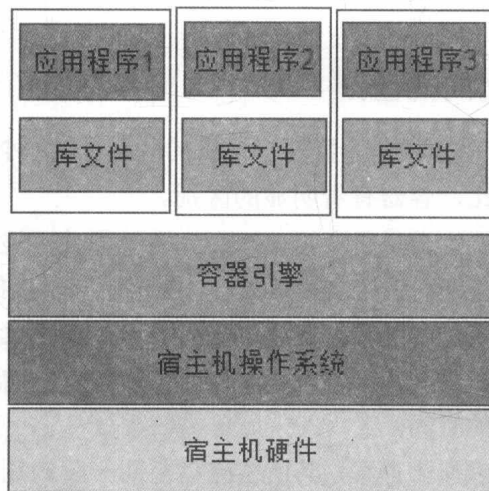
图 1-3 容器
