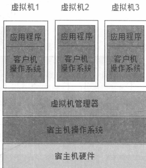
图 1-2 虚拟机
