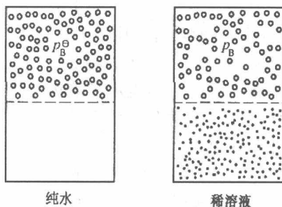
图1-3 纯水和稀溶液的蒸气压对比示意图
