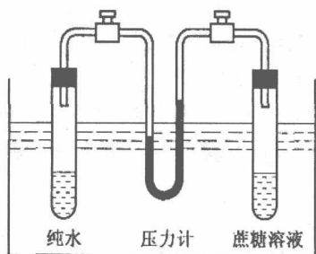
图1-2 非电解质稀溶液蒸气压下降示意图
