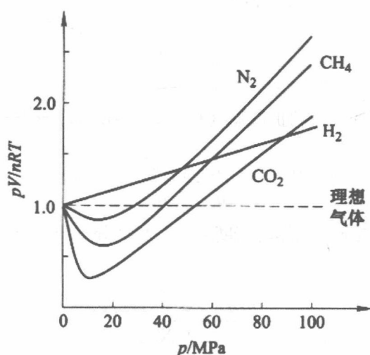
图1-1 几种气体的 pV/nRT-p (200K)
