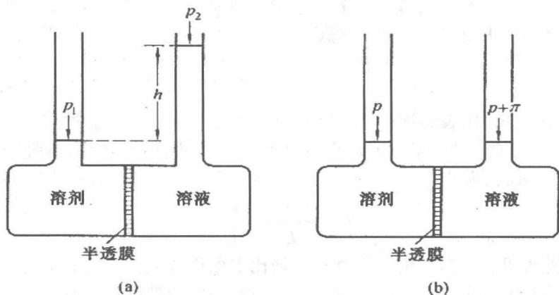
图1-5 渗透压示意图
