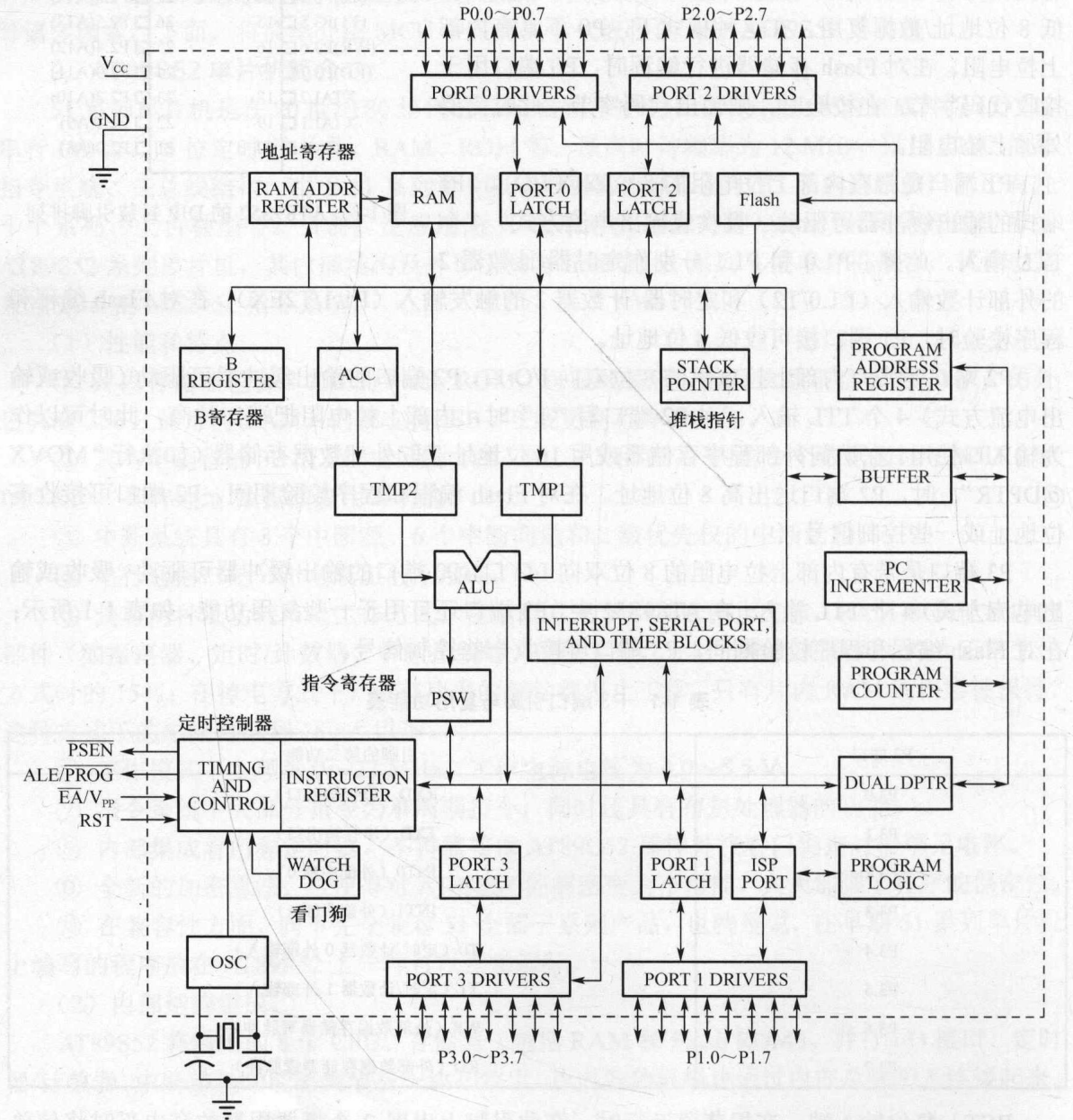
图 1-4 AT89S52 的结构框图
