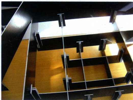
图 1-11 节点模型
