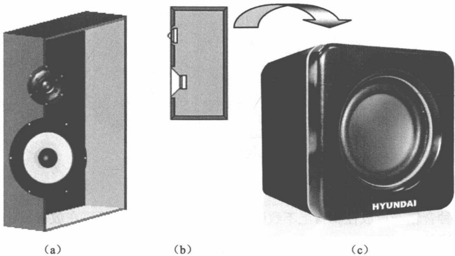
图 1-7 密闭式音箱
