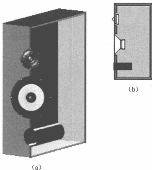
图 1-8 倒相式音箱结构图
