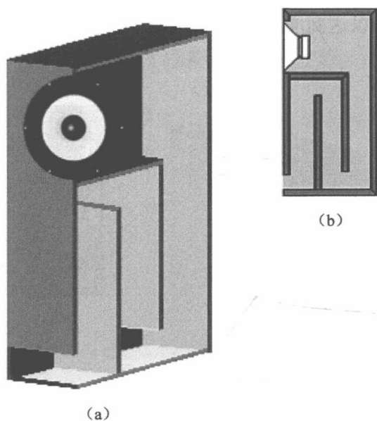
图 1-9 传输线式音箱
