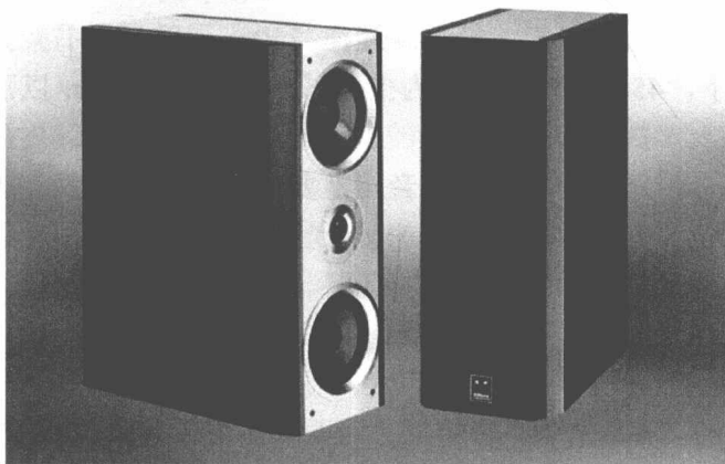
图 1-10 哑铃式音箱的箱体结构
