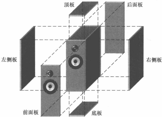
图 1-3 音箱示意图
