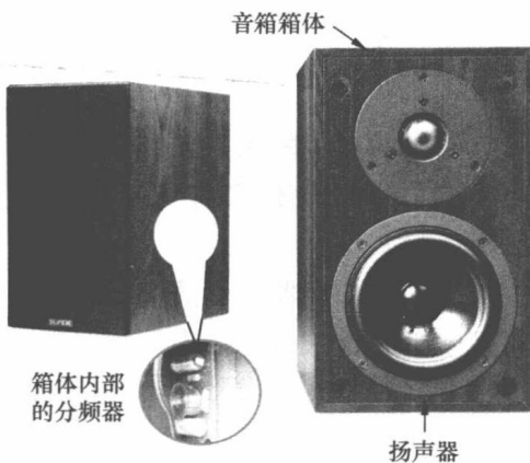
图 1-1 音箱的构成
