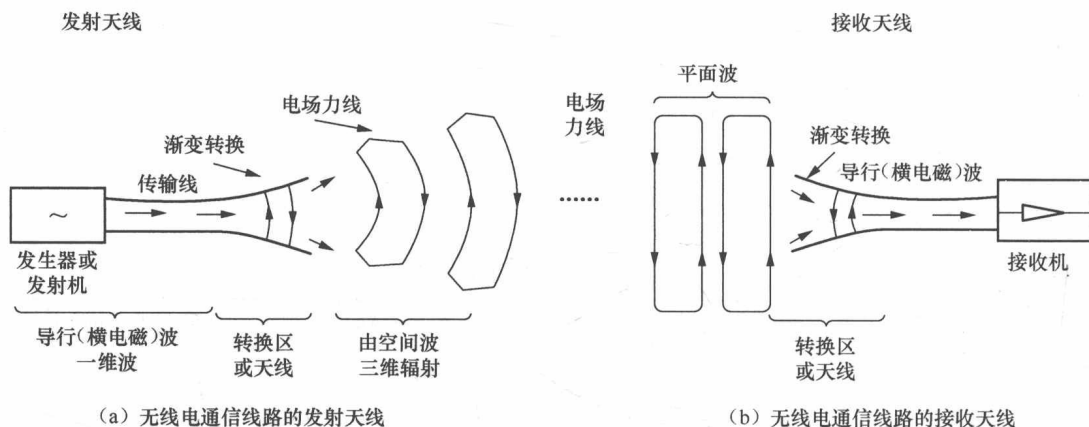
图 1.3.1 天线能量转换原理示意图
