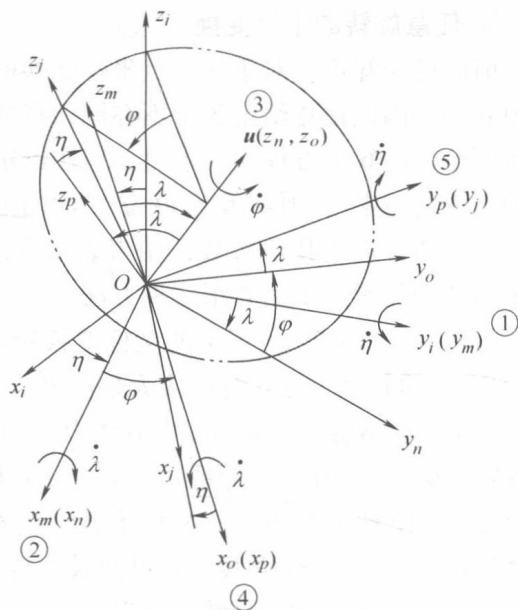
图 1-8 绕 u 轴旋转相当于五次坐标变换
