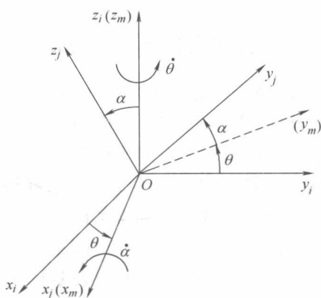
图 1-5 绕两个坐标轴旋转的坐标变换
