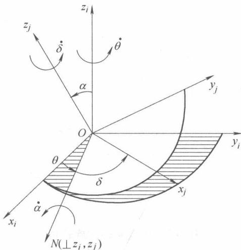
图 1-6 3 个欧拉角表示的坐标变换
