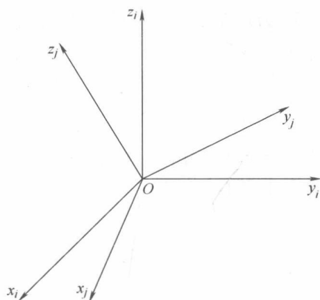
图 1-1 两个共原点的坐标系
