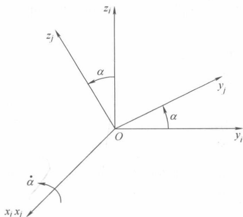
图 1-3 绕 x 轴旋转的坐标变换
