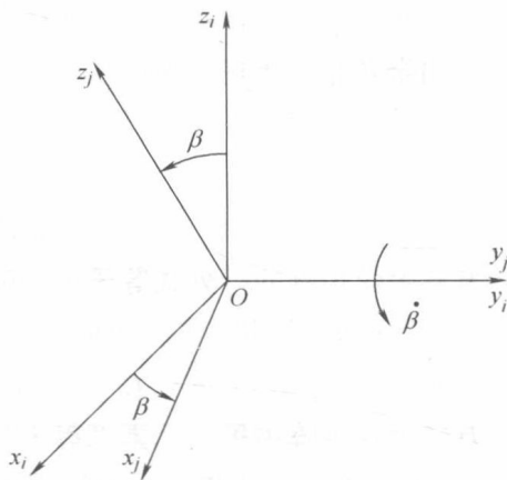
图 1-4 绕 y 轴旋转的坐标变换
