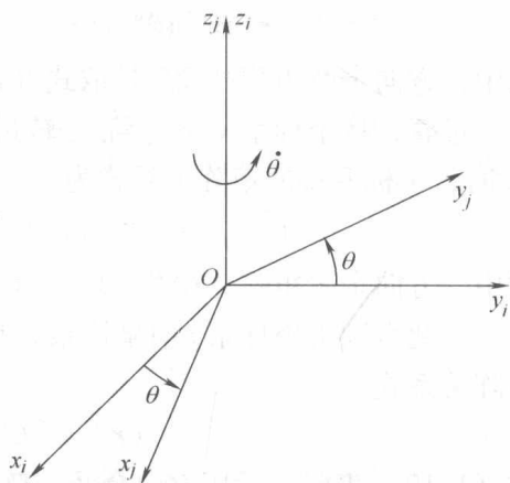
图 1-2 绕 z 轴旋转的坐标变换
