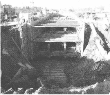
图 1.1-5 北京地铁基坑坍塌事故
