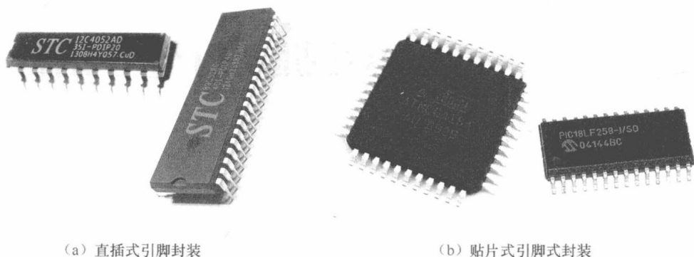
图1-2 几种常见单片机外形
