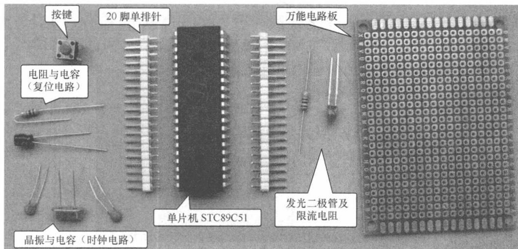
图1-6 一个按键控制一只发光二极管亮灭的单片机电路元件和万能电路板
