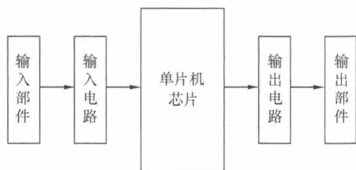
图1-3 典型的单片机应用系统的组成
