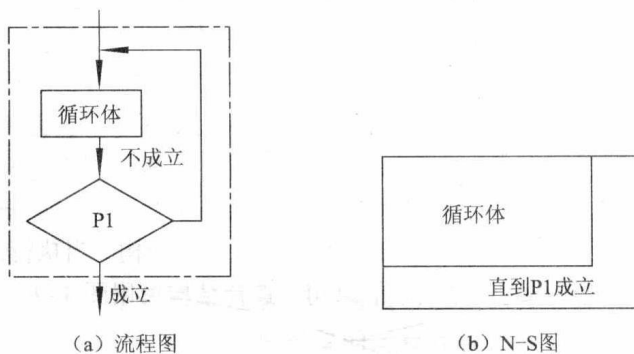
图 1-1-5 直到型循环结构
