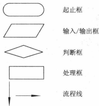
图 1-1-1 流程图符号
