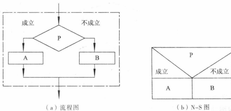
图 1-1-3 选择结构
