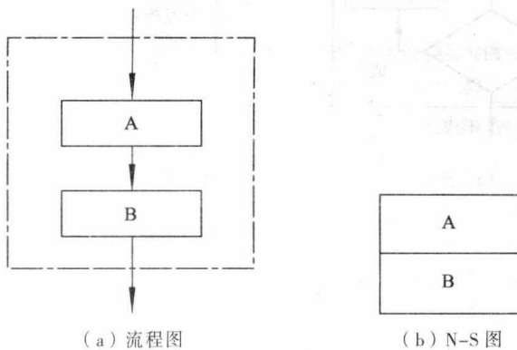
图 1-1-2 顺序结构
