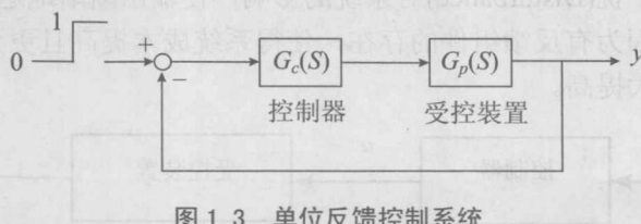
图 1.3 单位反馈控制系统
