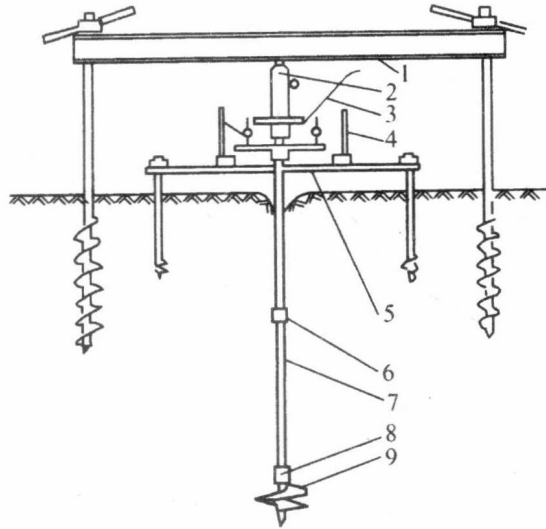
图 1-3 螺旋板载荷试验装置
