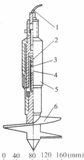
图 1-2 螺旋板结构示意图
