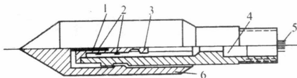
图 1-6 单桥探头结构
