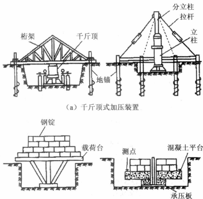
(a) 千斤顶式加压装置 (b) 载荷台式加压装置 图 1-1 静力载荷试验设备结构
