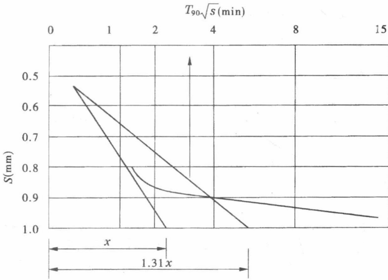
图 1-5 S\sqrt{t} 曲线
