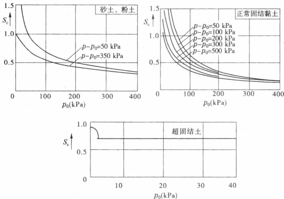
图 1-4 p_0-S_c 关系曲线
