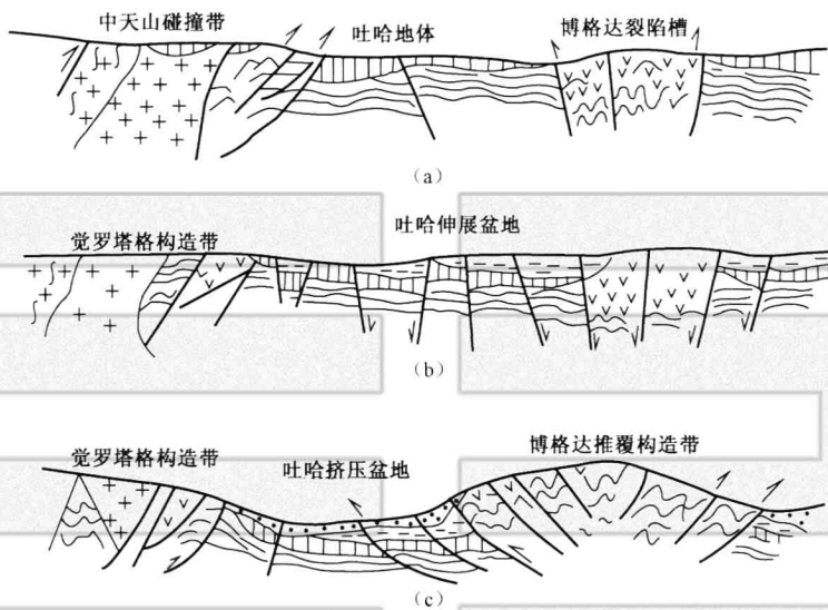
图 1-2 吐哈盆地构造演化示意图(据张鹏飞等,1997,修改)
