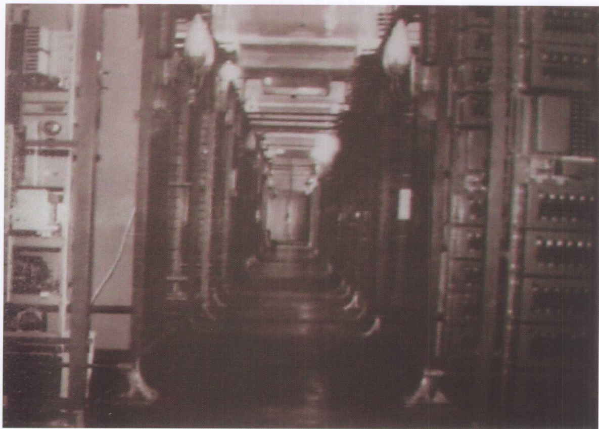
▲ 1961年，贵阳市正式投入使用的市话二分局JZB-1A交换机。
