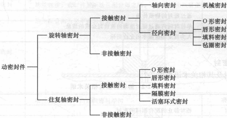
图 1-2 动密封件的分类
